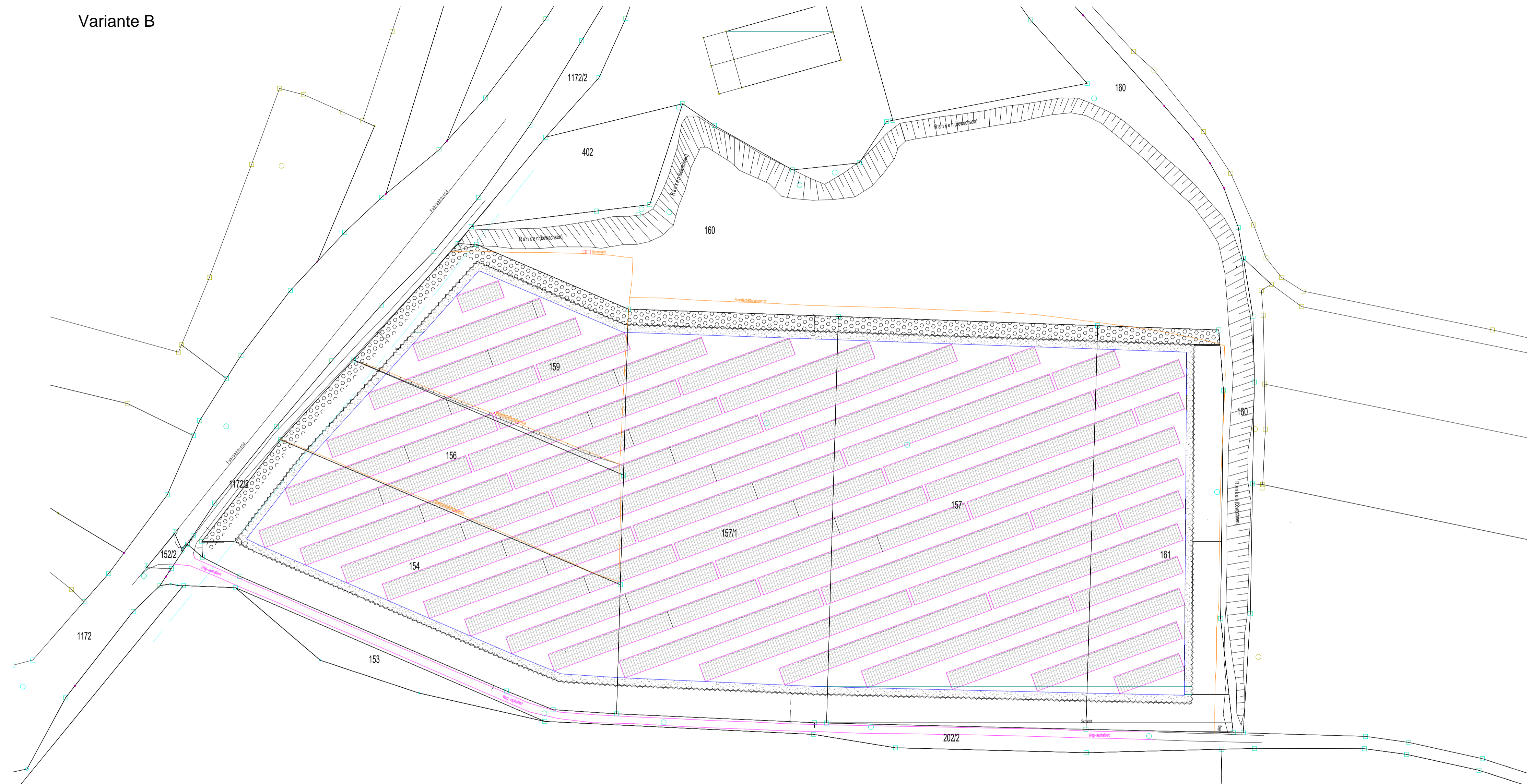
PV Freiflächenanlage "Engelbrechtsmünster III" Modulbelegung - Ausrichtung Südosten
